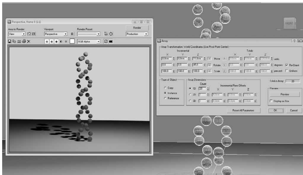
Obrázek 2.27. Šroubovice vytvořená nástrojem Array. Jde o kombinaci dvou transformací (posunutí a otočení) s využitím pouze 1D (druhé rameno šroubovice bylo vytvořeno stejně jako první, pouze s jinou počáteční pozicí první koule). Předpokladem správného výsledku je přemístění transformačního středu pivotu (gizma) koule, čehož docílíte přes panel Hierarchy → tlačítko Affect Pivot Only .
