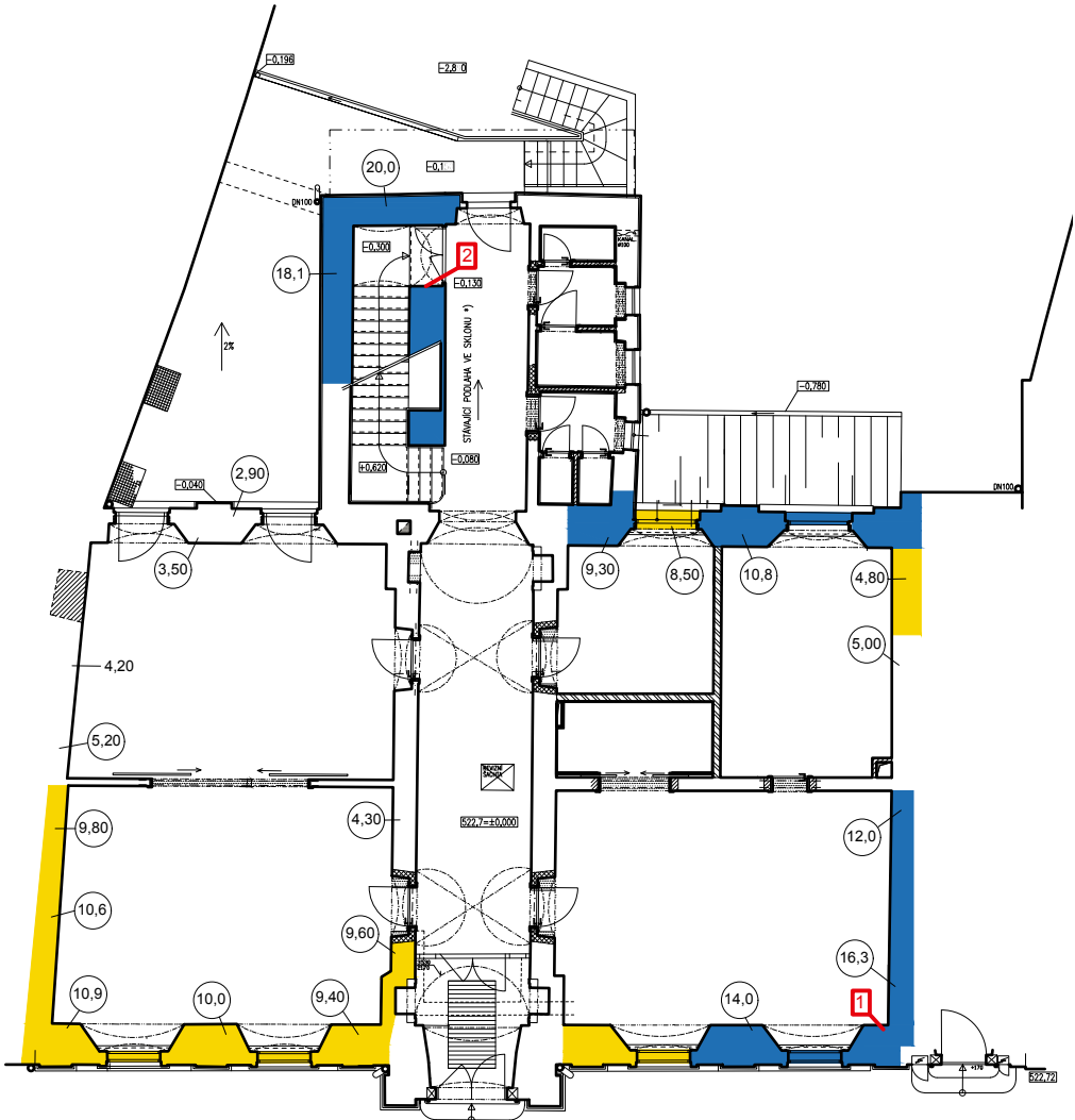
Obrázky 1, 2 Vyhodnocení stavu zdiva z hlediska vlhkosti u dispozičně složitěho památkově chráněného objektu.
