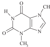
teobromin
