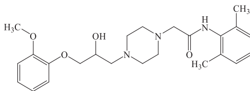
ranolazin
