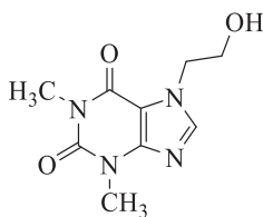
etofylin
