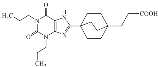
tonapofylin
