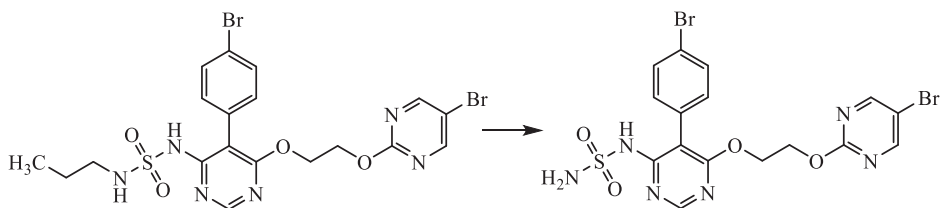
macitentan
