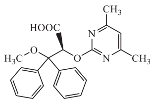
ambrisentan
