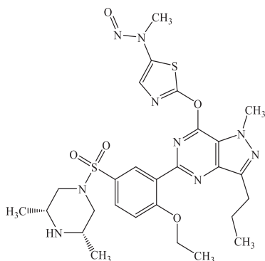
nitrosoprodinafil
