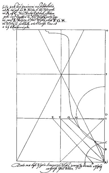
■ obrázek 3 Z „Návodu k liti a přípravě děl a kulí, hmoždírů, zvonů, vodotrysků...“, V. Kříčka z Bítvyšky
