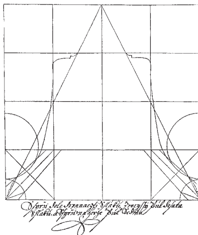
■ obrázek 2 Z „Návodu k liti a přípravě děl a kulí, hmoždírů, zvonů, vodotrysků...“, V. Kříčka z Bítvyšky
